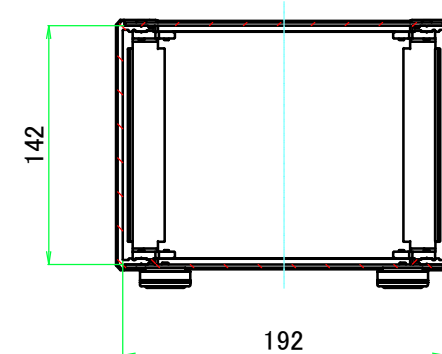
A-A ( 1 : 4.5 )
